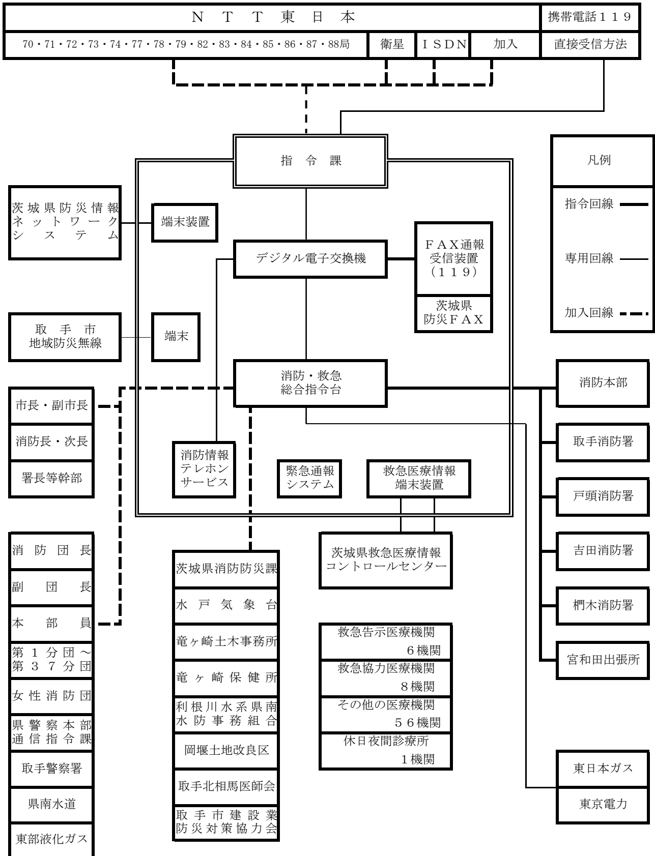
(1) 消防通信系統図
